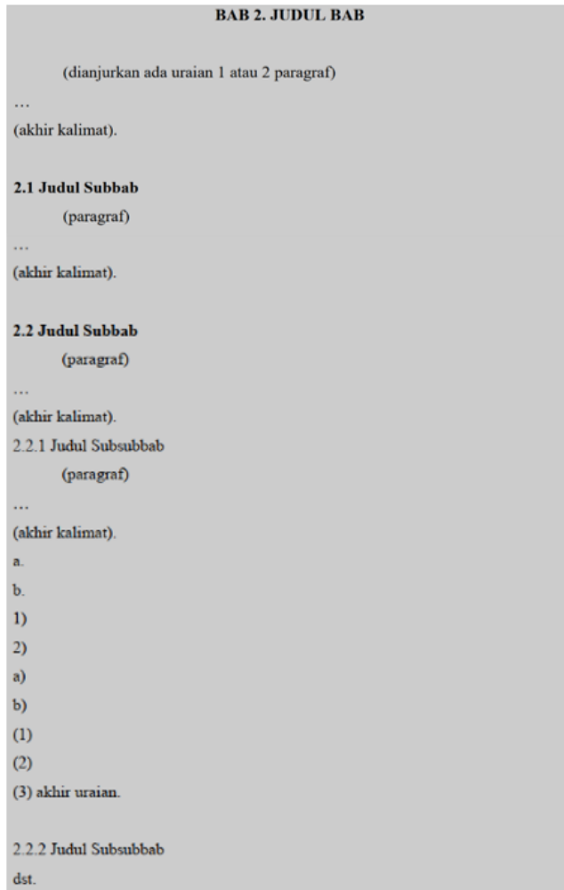
Gambar 53. Contoh Penomoran
